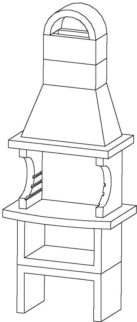
Termokamin Schema di montaggio Barbeque
